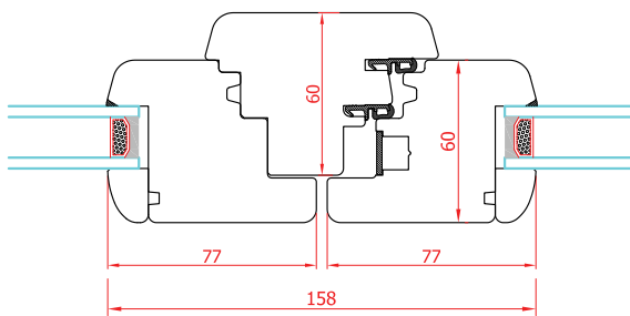
nodo centrale con montantino
