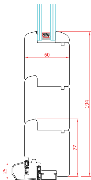
nodo inferiore soglia alluminio
