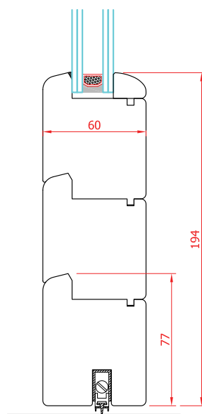
nodo inferiore parafreddo
