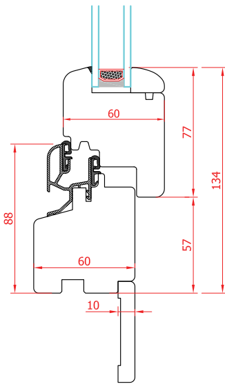
nodo inferiore gocciolatoio alluminio
