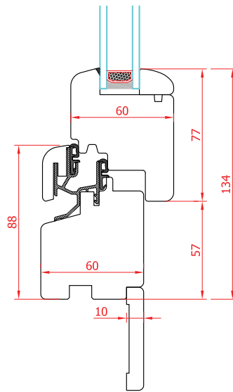
nodo inferiore gocciolatoio ricoperto
