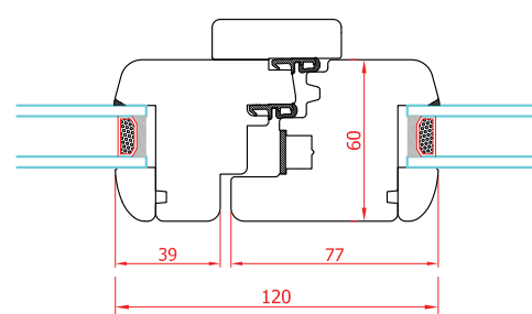
nodo centrale con scambio battuta
